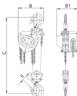
Pullmaster II 5000kg
