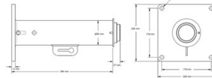
Abmessungen der Art.-Nr. 5BP5
