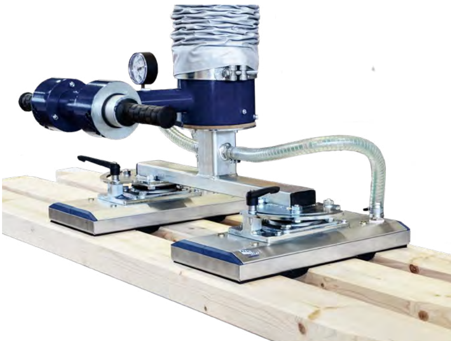
Der VUSS-Flächengreifer ermöglicht problemloses Handling von unebenen, strukturierten Oberflächen sowie bei undefinierten Aufnahmesituationen oder unterschiedlichen Abmessungen.
