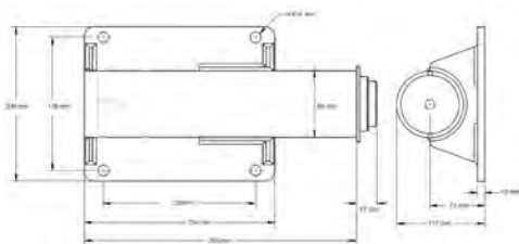
Abmessungen der Art.-Nr. 5BW5
