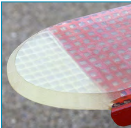
secutex-Zinkenschutz SZ-S1 Standardausführung mit flexibler Spitze
