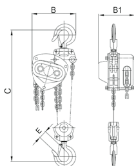
Pullmaster II 500kg
