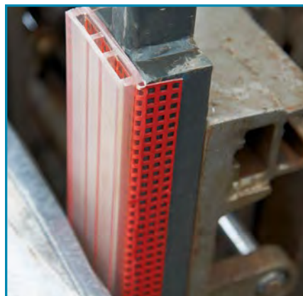
secutex-Gabelrückenschutz SZ-S2 Hohlprofil Robust mit hohem Dämpfungseffekt
